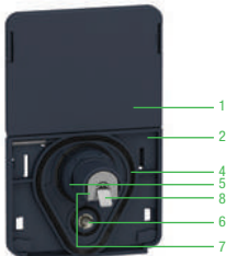
VW3A1112 Arka yüzü
