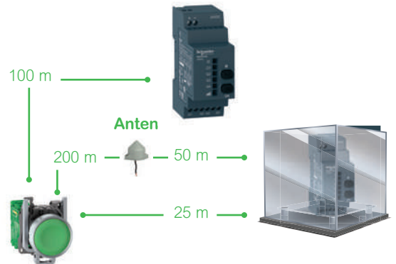
Metal Kabin İçerisindeki Alıcı
